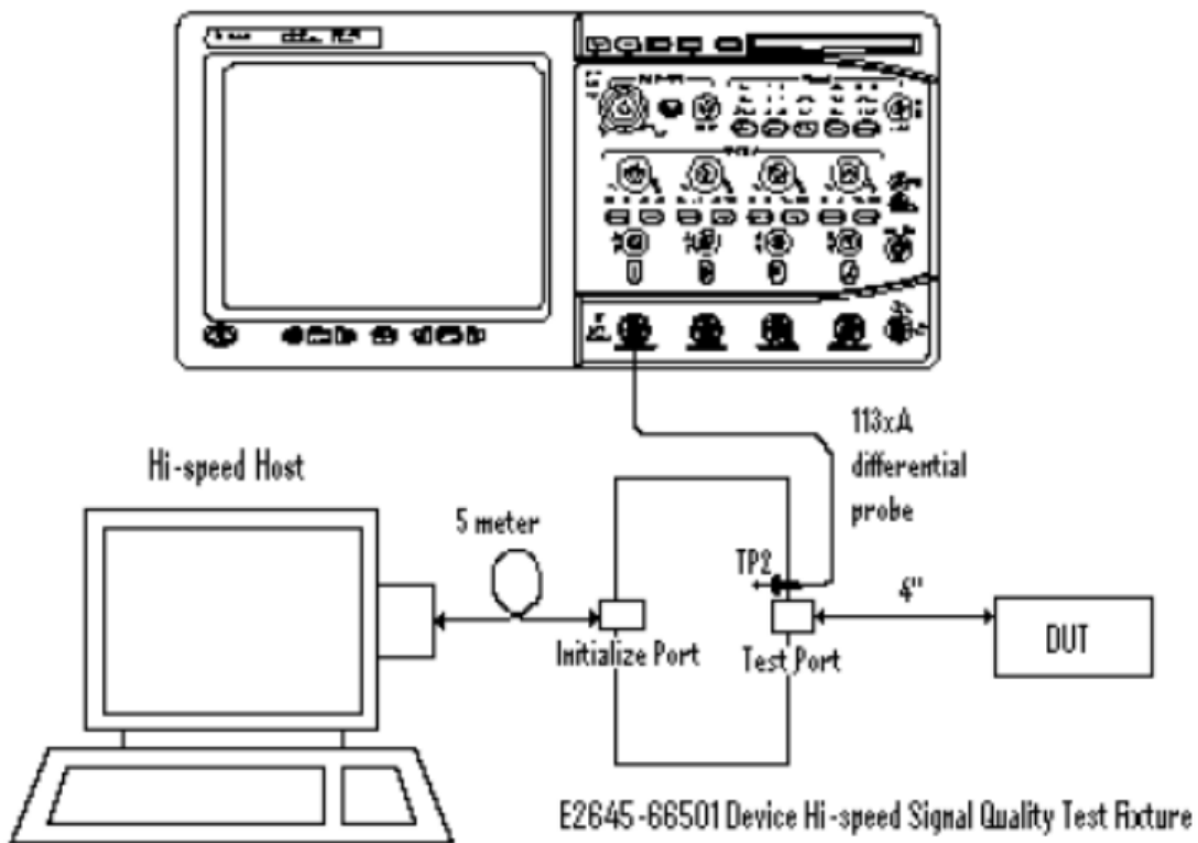
图 1-4 Agilent USB 2.0 SQ 测试环境
