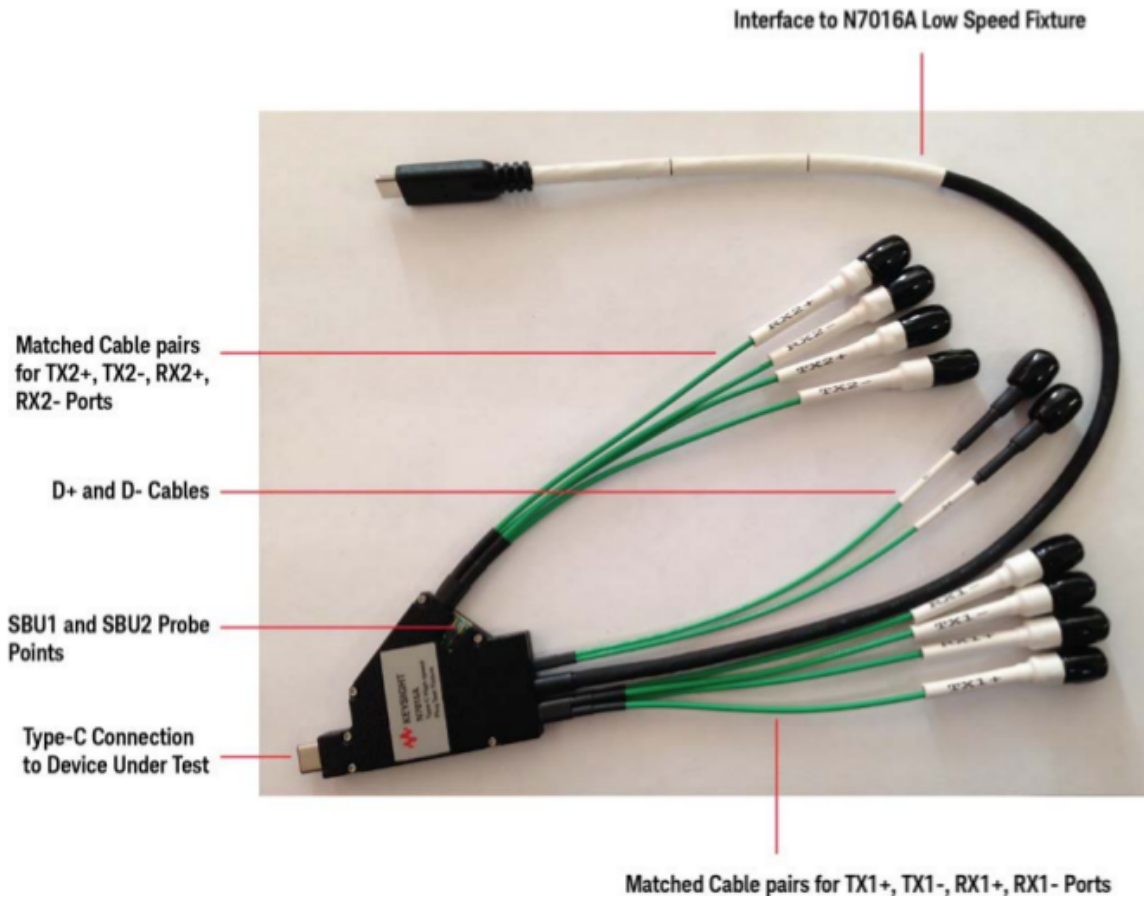
图 3-9 Agilent USB 3.0 Type-C 测试夹具 N7015A
