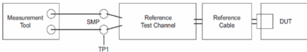
图 3-2 USB 3.0 Tx 测试模型
