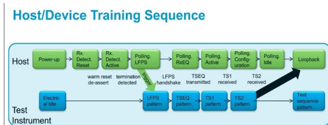
图 3-25 USB 3.0 进入 Loopback mode 的流程
