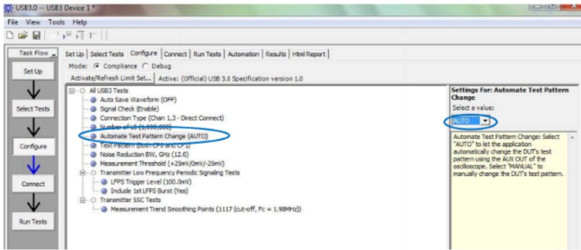
图 3-14 USB 3.0 Device Tx 测试条件设置
