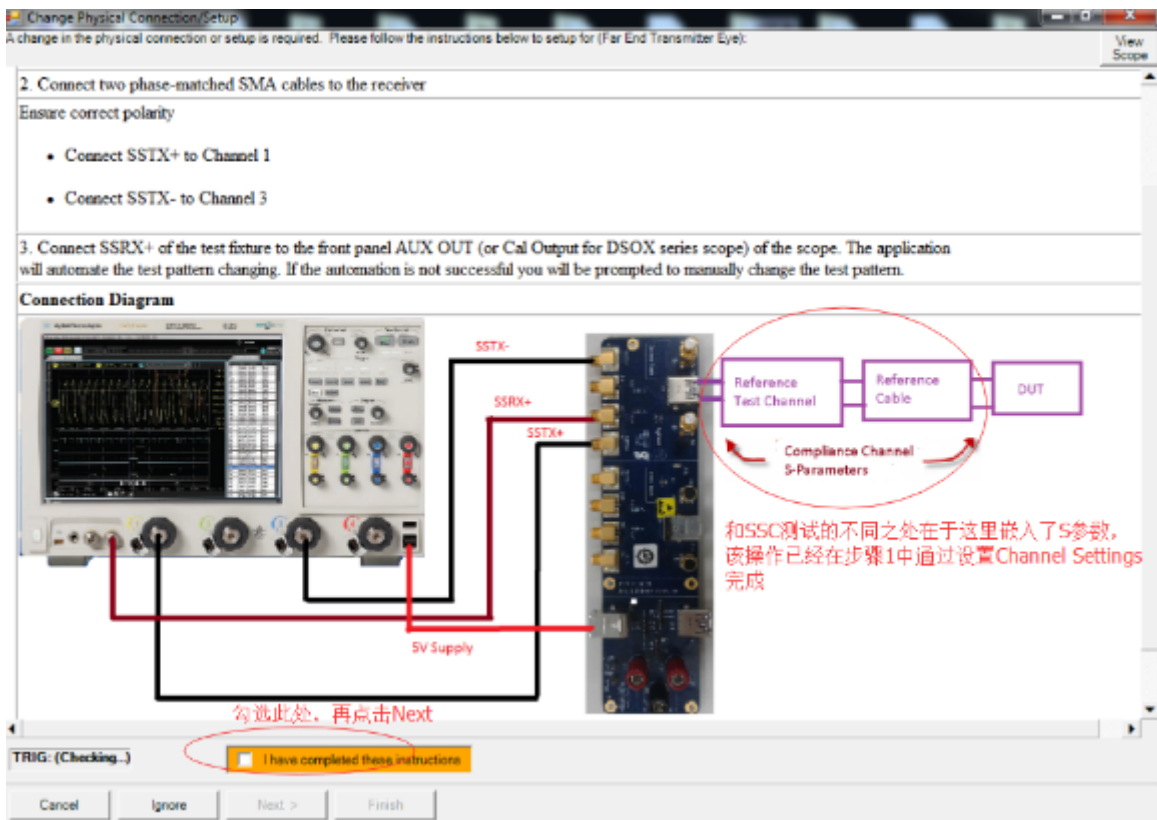
图 3-19 USB 3.0 Device Tx 眼图及抖动测试
