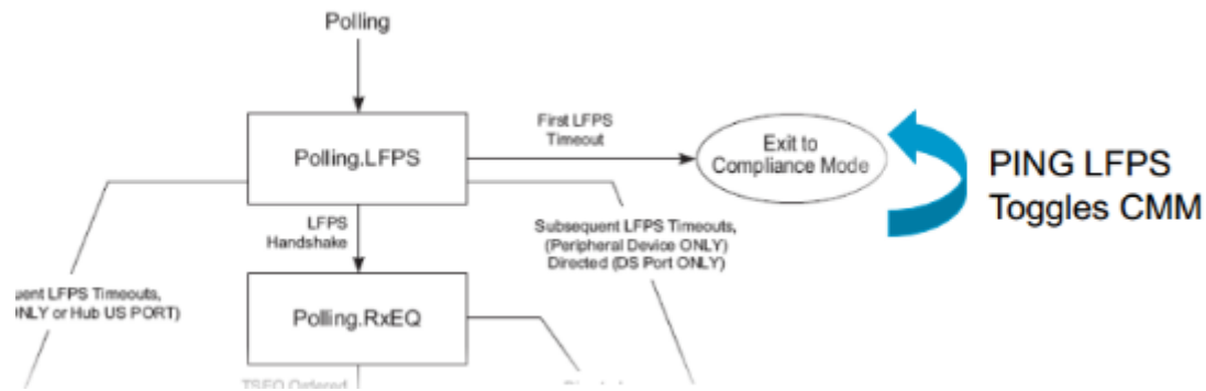
图 3-6 USB 3.0 进入 Compliance Mode 的流程
