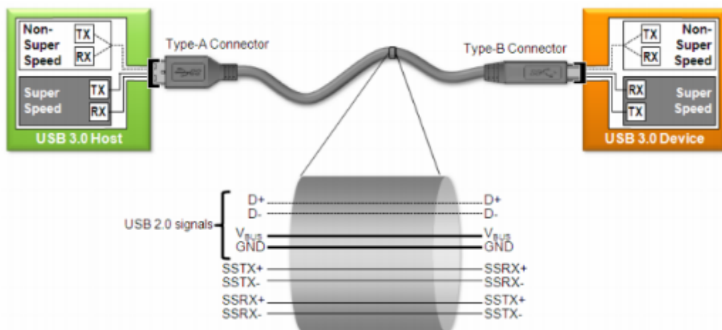
图 3-1 USB 3.0 总线架构
